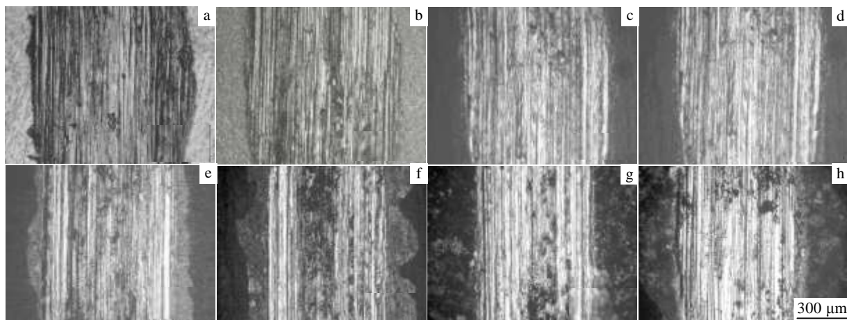
图 6 Ti6Al4V 和不同温度热氧化层的磨痕
