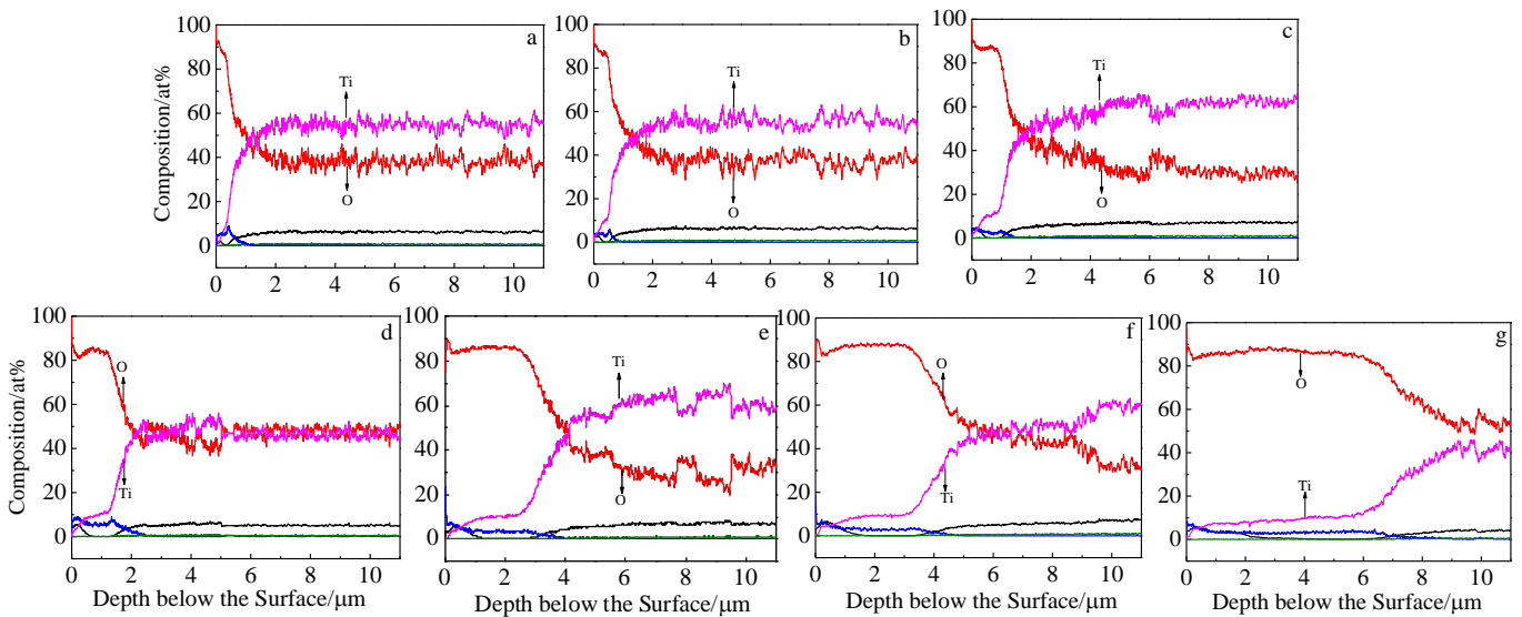
图2 不同温度下 Ti6Al4V 表面热氧化层的成分分布曲线 Fig.2 Composition distributions of thermal oxidation layers on Ti6Al4V alloy obtained at different temperatures: (a) 873 K, (b) 898 K, (c) 923 K, (d) 948 K, (e) 973 K, (f) 998 K, and (g) 1023 K
