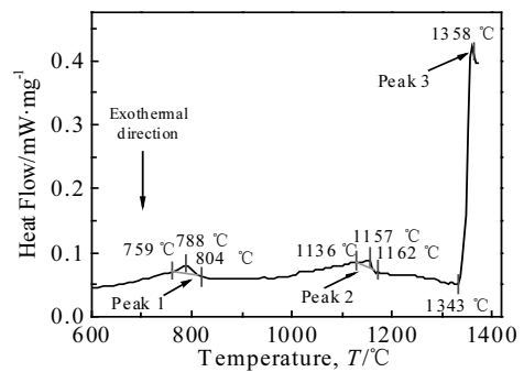
图 6 Co-9Al-3W-30Ni-2Ta-3.5Ti 合金的 DSC 升温曲线
