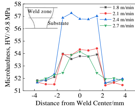
图 13 焊接接头显微硬度随焊缝中心距离的变化
