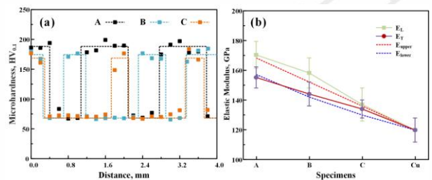
图 6 Cu/316L 复合材料的 (a) 显微硬度和 (b) 弹性模量
