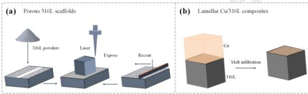
图 1 复合材料制备过程示意图：(a) SLM 制备多孔 316L 骨架，(b) 熔体浸渗获得 Cu/316L 复合材料
