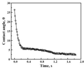
图 3 1100^\circ\text{C} ( <5 \times 10^{-4}\text{ Pa} ) Cu-316L 接触角-时间曲线
