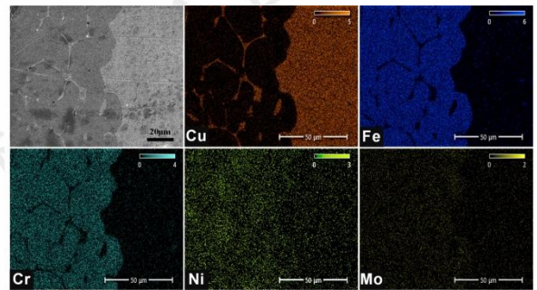
图 5 Cu/316L 界面的扫描图及元素分布
