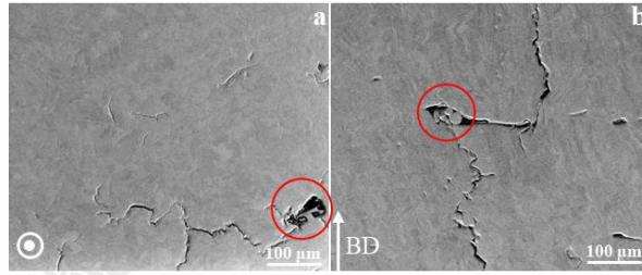
图 8 W-25Re 合金试样内部缺陷的 SEM (18# 575 J/mm 3 )
