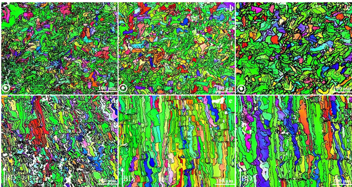
图 9 W-25Re 合金试样的 IPF 图
