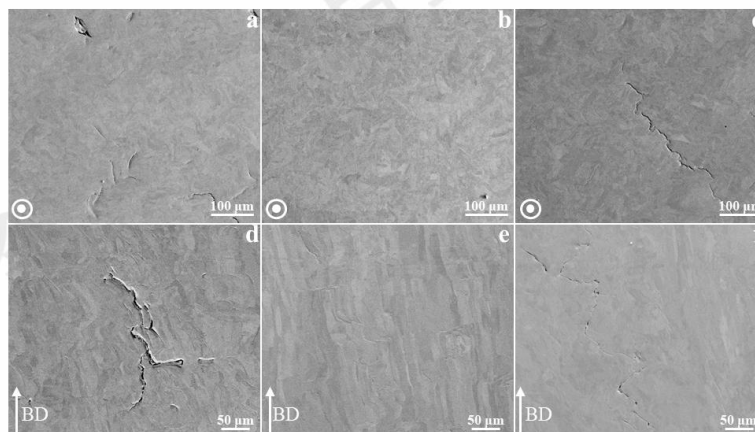
图 7 不同工艺参数条件下制备 W-25Re 合金试样的 SEM
