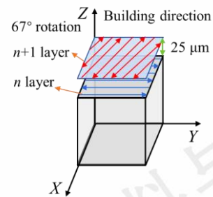
图 2 扫描策略示意图
