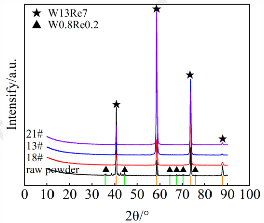
图 11 W-25Re 合金原料粉末和试样 XRD
