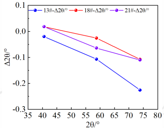
图 12 W-25Re 原料粉末和合金试样 \Delta 2\theta 的变化
