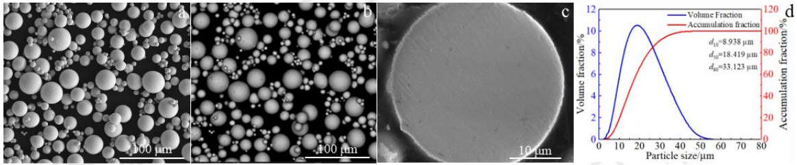
图 1 球形 W-25Re 合金粉末检测结果
