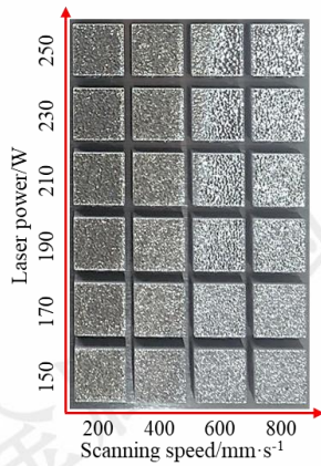
图3 不同工艺参数条件下的 W-25Re 合金试样
