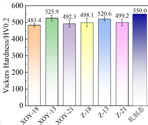
图 13 W-25Re 合金试样显微维氏硬度
