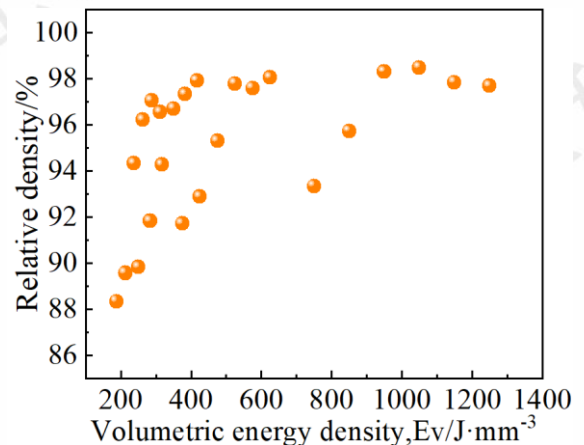
图6 不同体能量密度条件下 W-25Re 合金试样的相对密度
