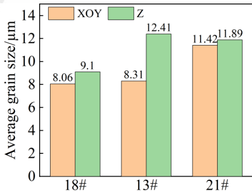
图 10 W-25Re 合金试样的平均晶粒
