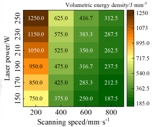
图5 不同工艺参数条件下的体能量密度值
