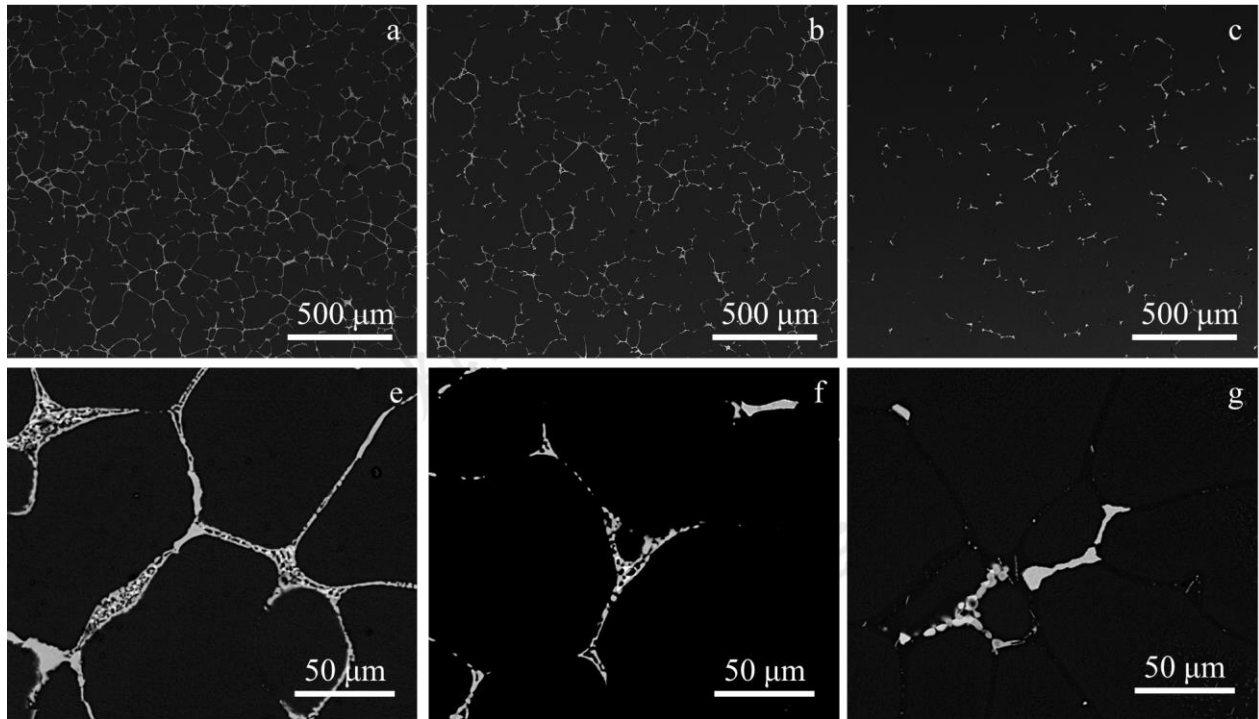
图 4 2024 铝合金在不同均匀化温度下保温 24 h 的 BSE 照片
