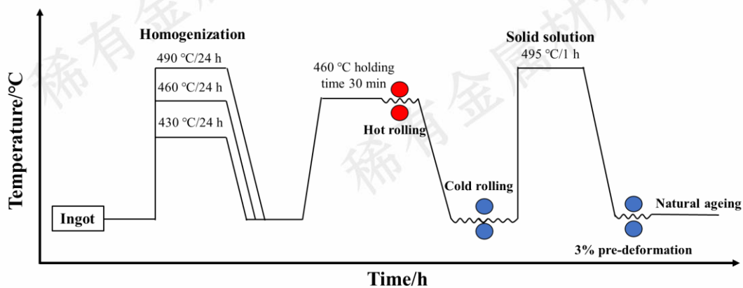
图 1 三组 2024-T3 板材的工艺流程图
