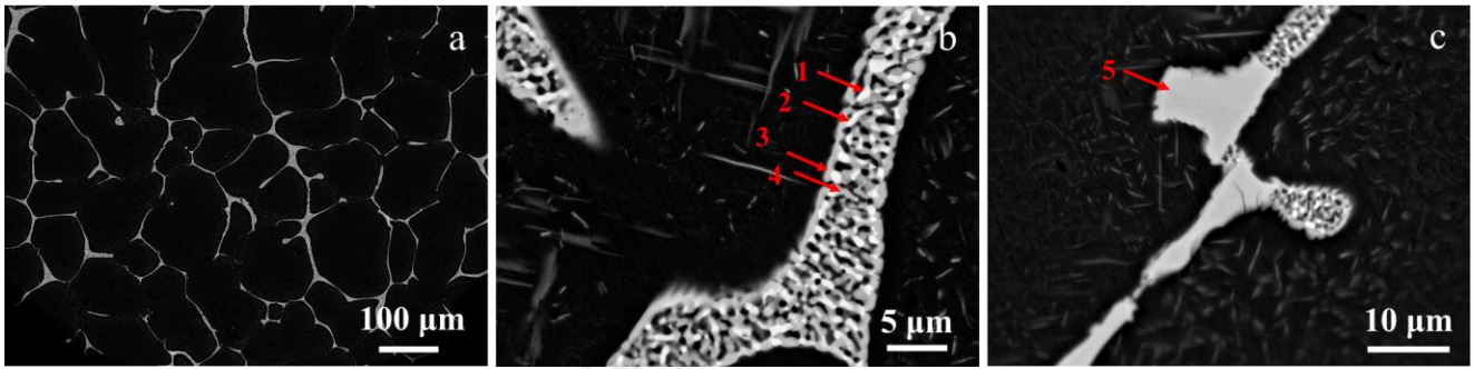
图 2 2024 合金铸锭的 BSE 图片
