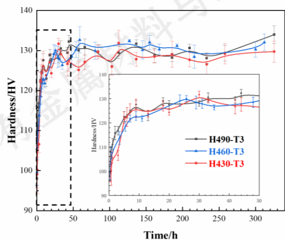
图 10 三组合金的自然时效硬化曲线
