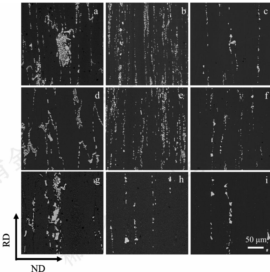
图 5 三组合金在不同状态下的 BSE 图片
