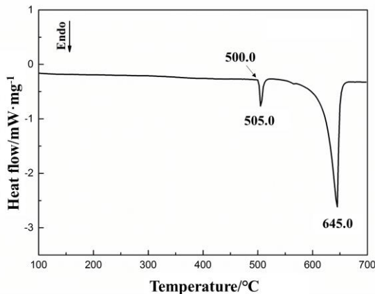
图 3 2024 合金铸锭的 DSC 曲线图
