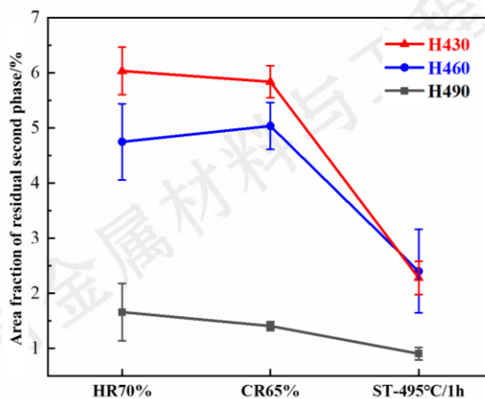
图 6 三组合金在不同阶段的残留第二相面积分数
