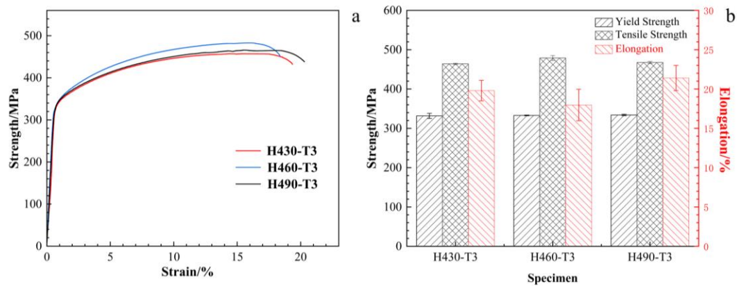
图 11 三组合金自然时效 7 天后 T3 态 2024 合金的室温拉伸性能
