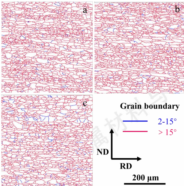
图 7 固溶淬火态合金 RD-ND 面的 GB 图
