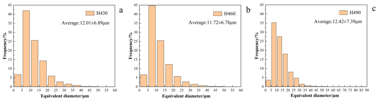
图 8 三组固溶淬火态合金的等效圆直径尺寸频率分布图
