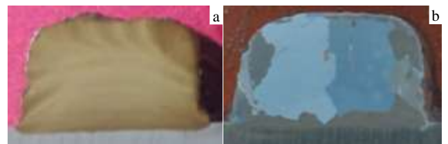
图 7 沉积态和标准热处理后 LSF 成形试样的宏观照片
