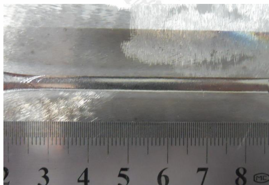
图 15 焊接接头的宏观形貌
