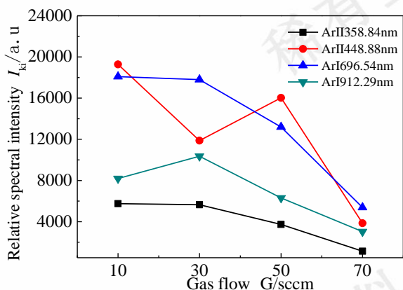
图 7 气体流量对空心阴极真空电弧光谱强度的影响
