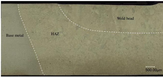
图 10 TC4 空心阴极真空电弧焊接接头的宏观组织形貌
