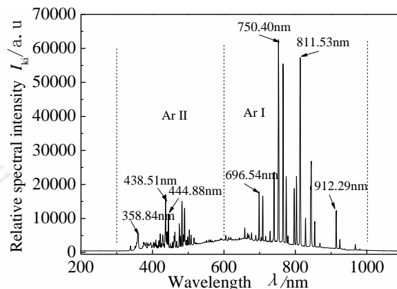
图5 空心阴极真空电弧光谱图
