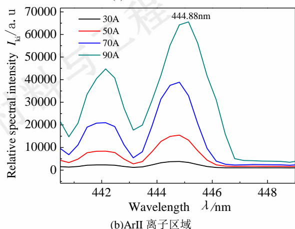
图 8 不同电流下空心阴极真空电弧光谱
