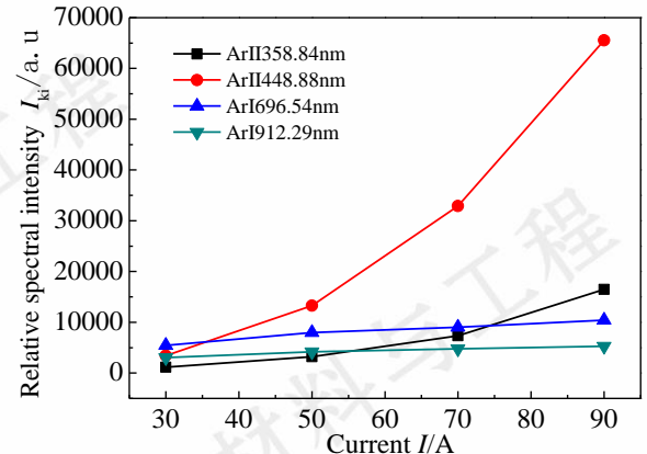
图 9 电流对空心阴极真空电弧光谱强度的影响
