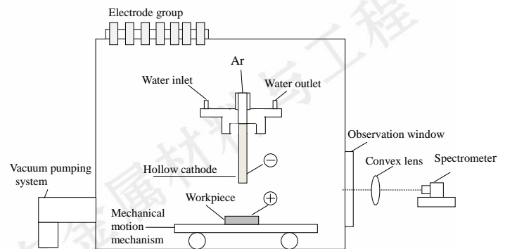
图 1 焊接实验系统示意图
