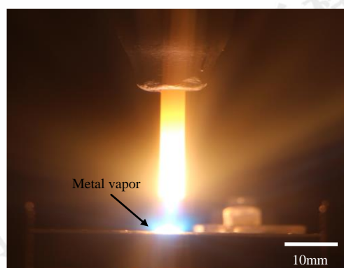
图 3 TC4 钛合金焊接过程的电弧形貌
