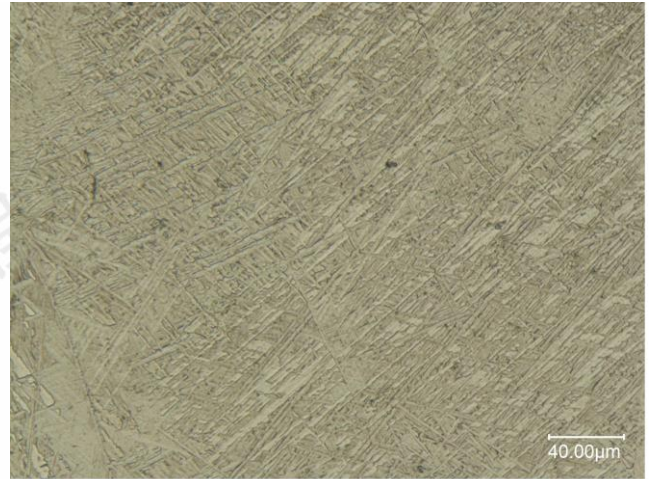
图 12 焊缝的显微组织
