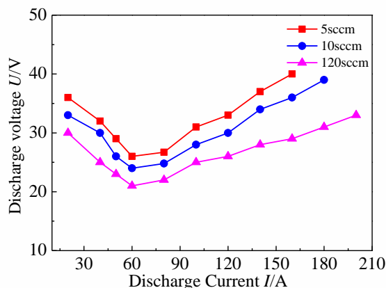
图 2 空心阴极真空电弧伏安特性曲线
