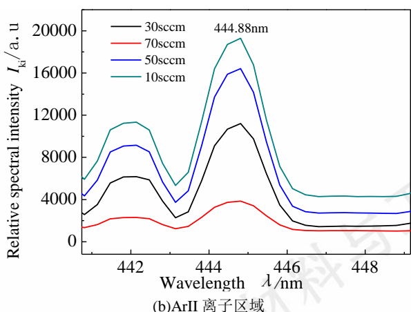
图 6 不同气体流量下空心阴极真空电弧光谱
