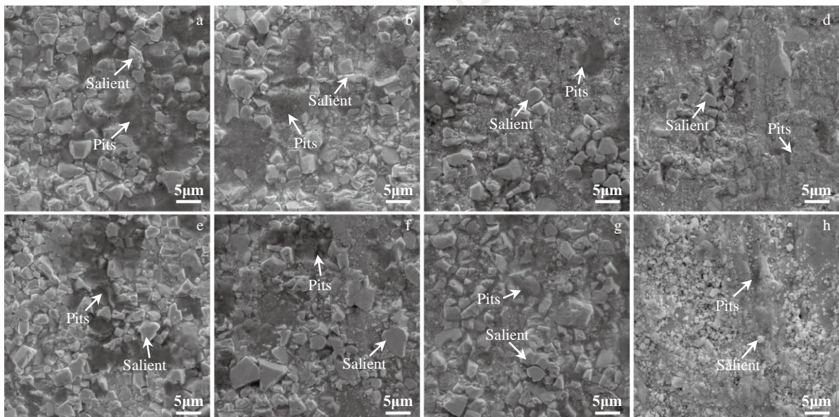
图 10 不同粘结相含量 WC-Co 和 WC-Ni-Fe 硬质合金磨损面的扫描电镜照片
