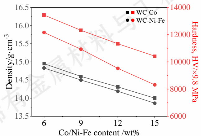
图4 不同粘结相含量WC-Co和WC-Ni-Fe硬质合金的密度与硬度
