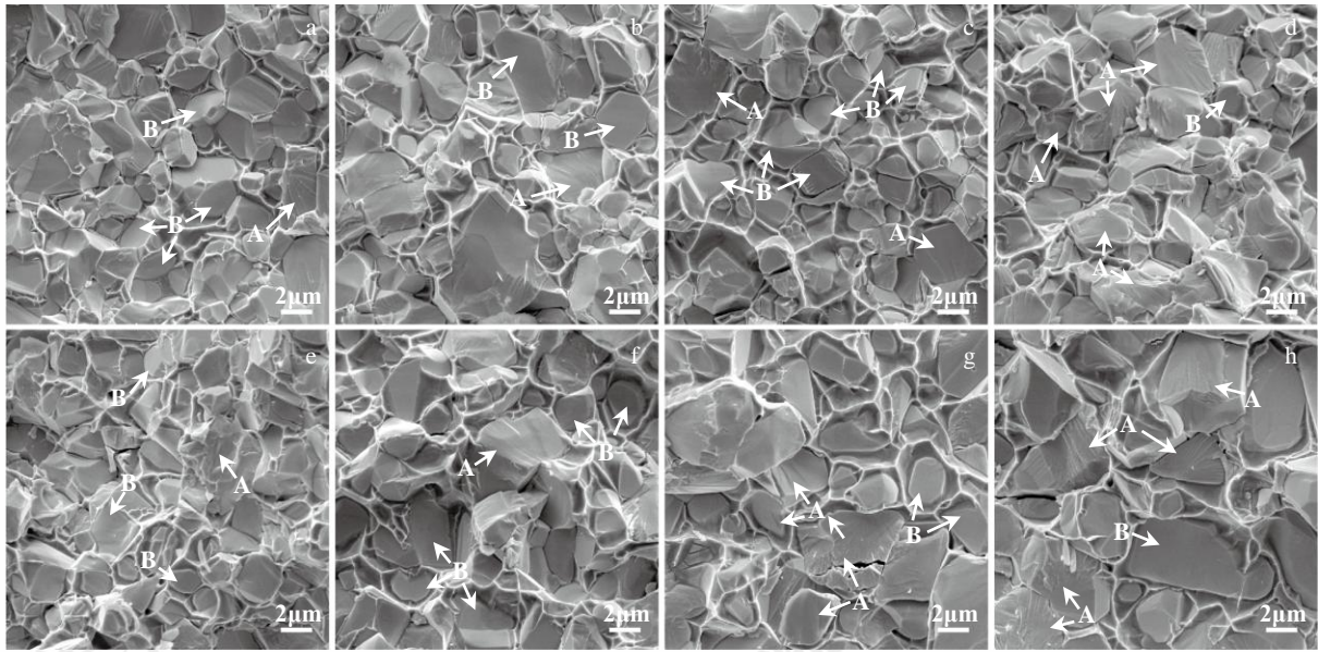
图 7 不同粘结相含量 WC-Co 和 WC-Ni-Fe 硬质合金的弯曲断口的 SEM 形貌
