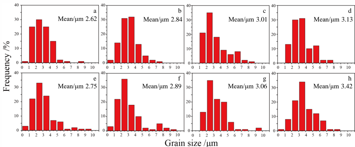
图3 不同粘结相含量 WC-Co 和 WC-Ni-Fe 硬质合金的晶粒尺寸
