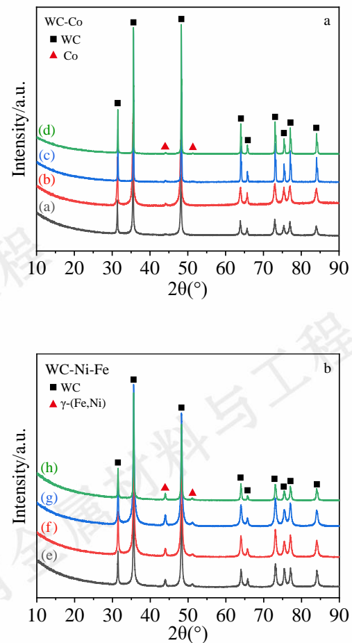
图 1 不同粘结相含量 WC-Co 和 WC-Ni-Fe 硬质合金的 XRD 图谱 Fig.1 XRD patterns of WC-Co and WC-Ni-Fe cemented carbides with different binder phase contents (a)WC-Co, (b)WC-Ni-Fe
