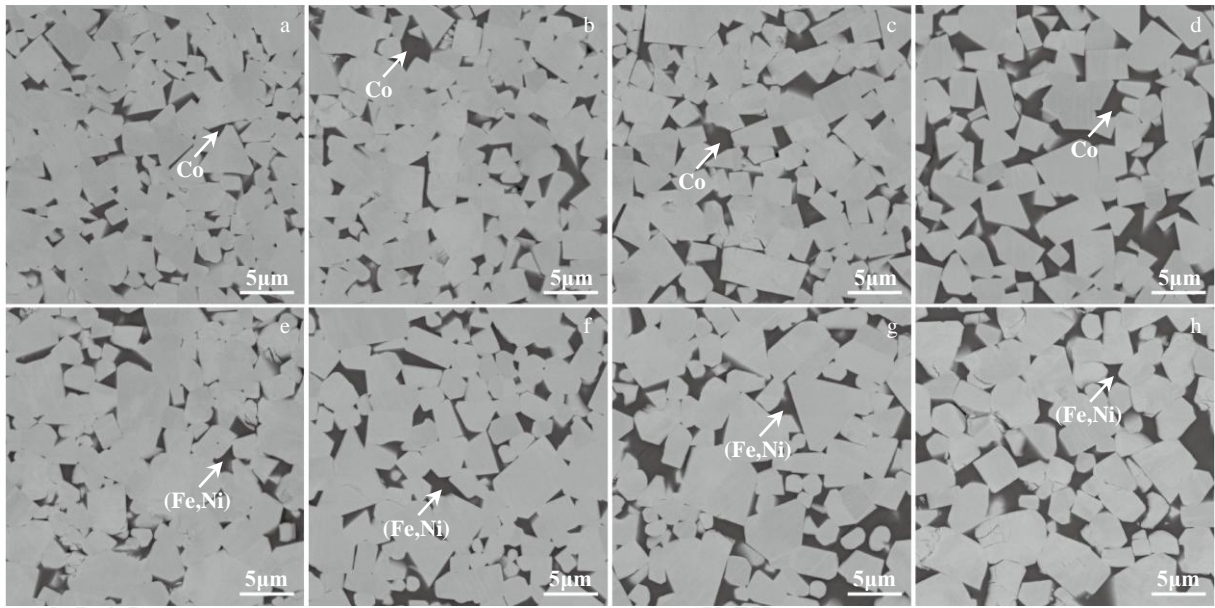
图2 不同粘结相含量 WC-Co 和 WC-Ni-Fe 硬质合金的扫描电镜照片
