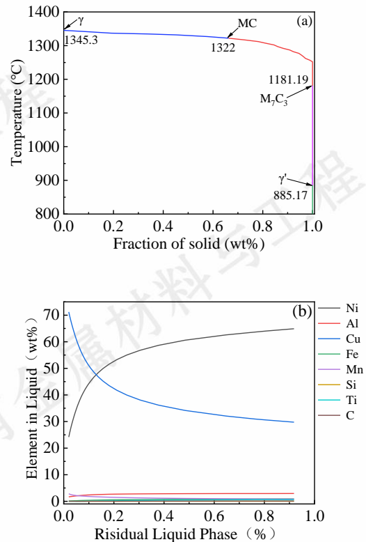
图2 (a) Monel K-500 合金凝固路径; (b) 凝固过程中元素再分配情况
