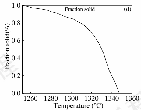
图4 Monel K-500 合金热物性参数: (a) 热导率-温度曲线; (b) 密度-温度曲线; (c) 热焓-温度曲线; (d) 固相百分数-温度曲线
