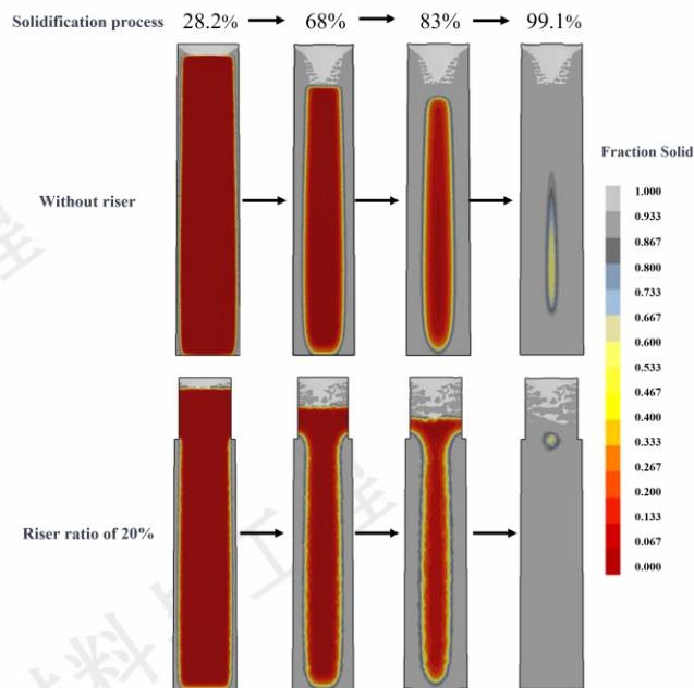
图8 不同冒容比 Monel K-500 合金真空感应锭凝固进程图
