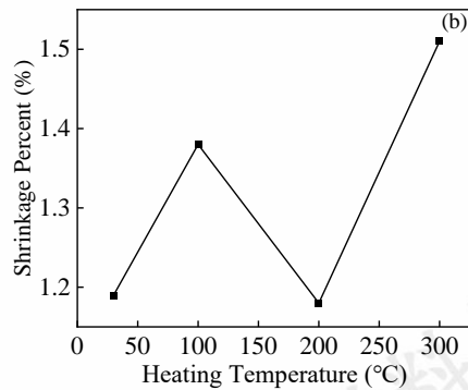
图11 (a) 6t Monel k-500 合金不同模具烘烤温度真空感应锭缩孔云图; (b) 6t Monel k-500 合金真空感应锭缩孔缺陷随模具烘烤温度变化图
