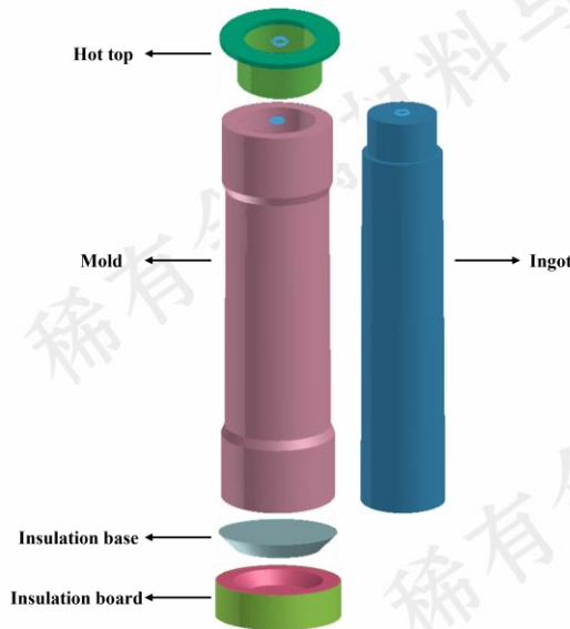
图3 Monel K-500 合金浇注系统几何模型
