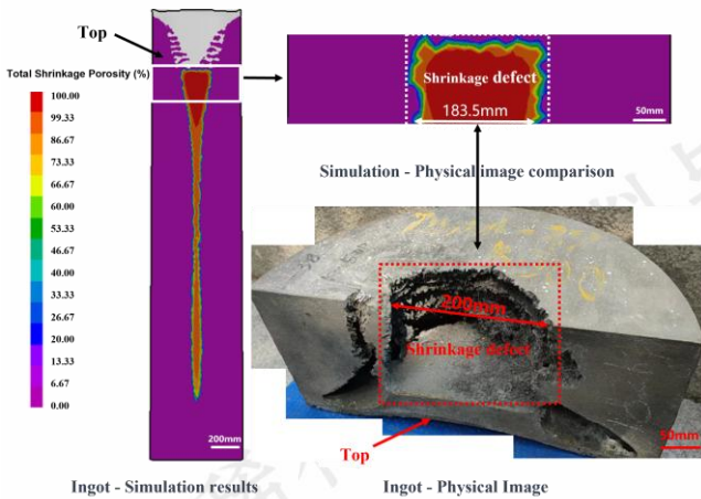
图6 Monel K-500 合金真空感应锭实物及模拟对照图
