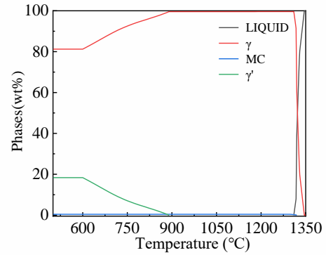
图1 MonelK-500 合金平衡相图
