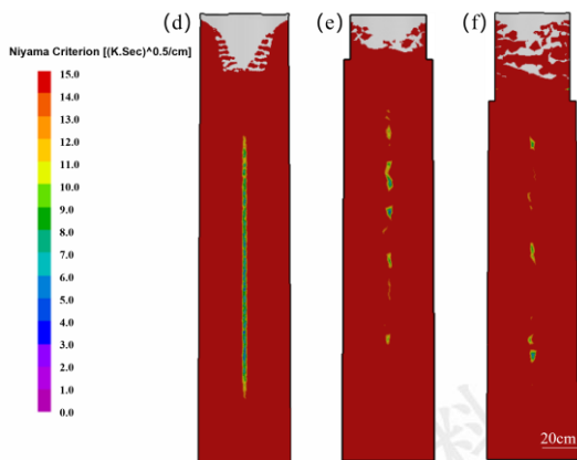
图7 6t 不同冒容比 Monel K-500 合金真空感应锭缩孔及 Niyama 判据云图 (a)、(d) 无冒口; (b)、(e) 冒容比为 10%; (c)、(f) 冒容比为 20%
