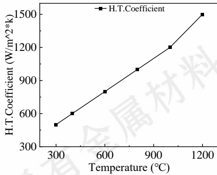
图5 Monel K-500 合金铸锭与铸锭模间对流换热系数曲线 [21]
